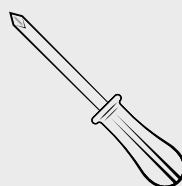
Tournevis
