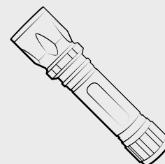
Torche
