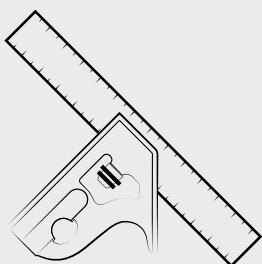
Équerre combinée
